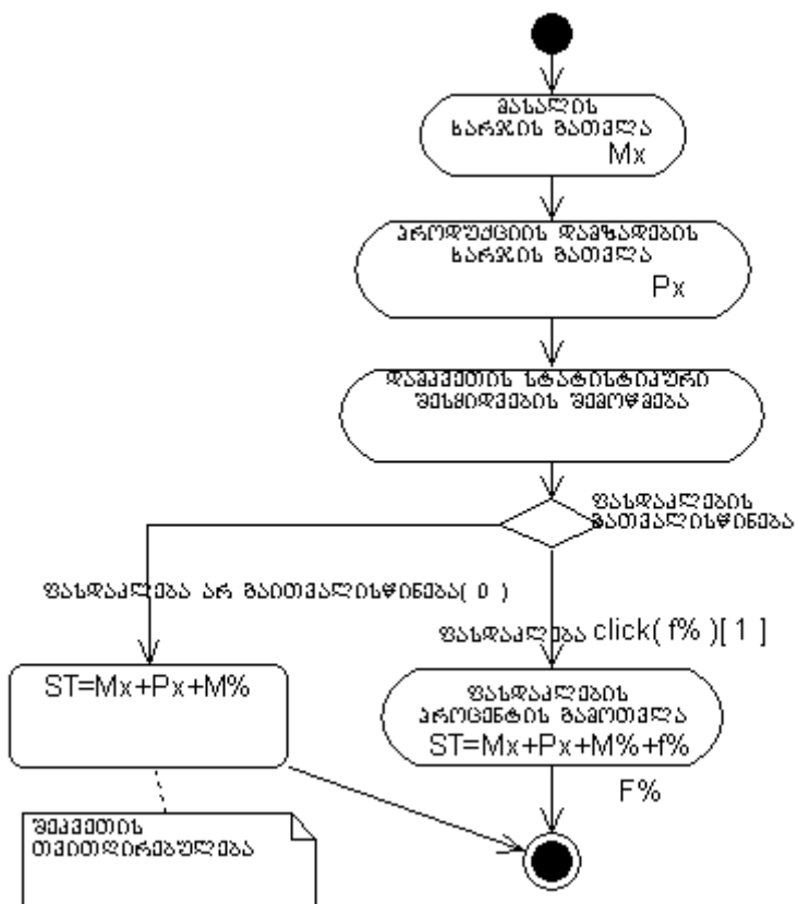
სურ. 4.11. შეკვეთის ფასის ფორმირების ქვედიაგრამის ფრაგმენტი პრეცედენტისთვის - პროლუქციის პარამეტრების დამუშავება
