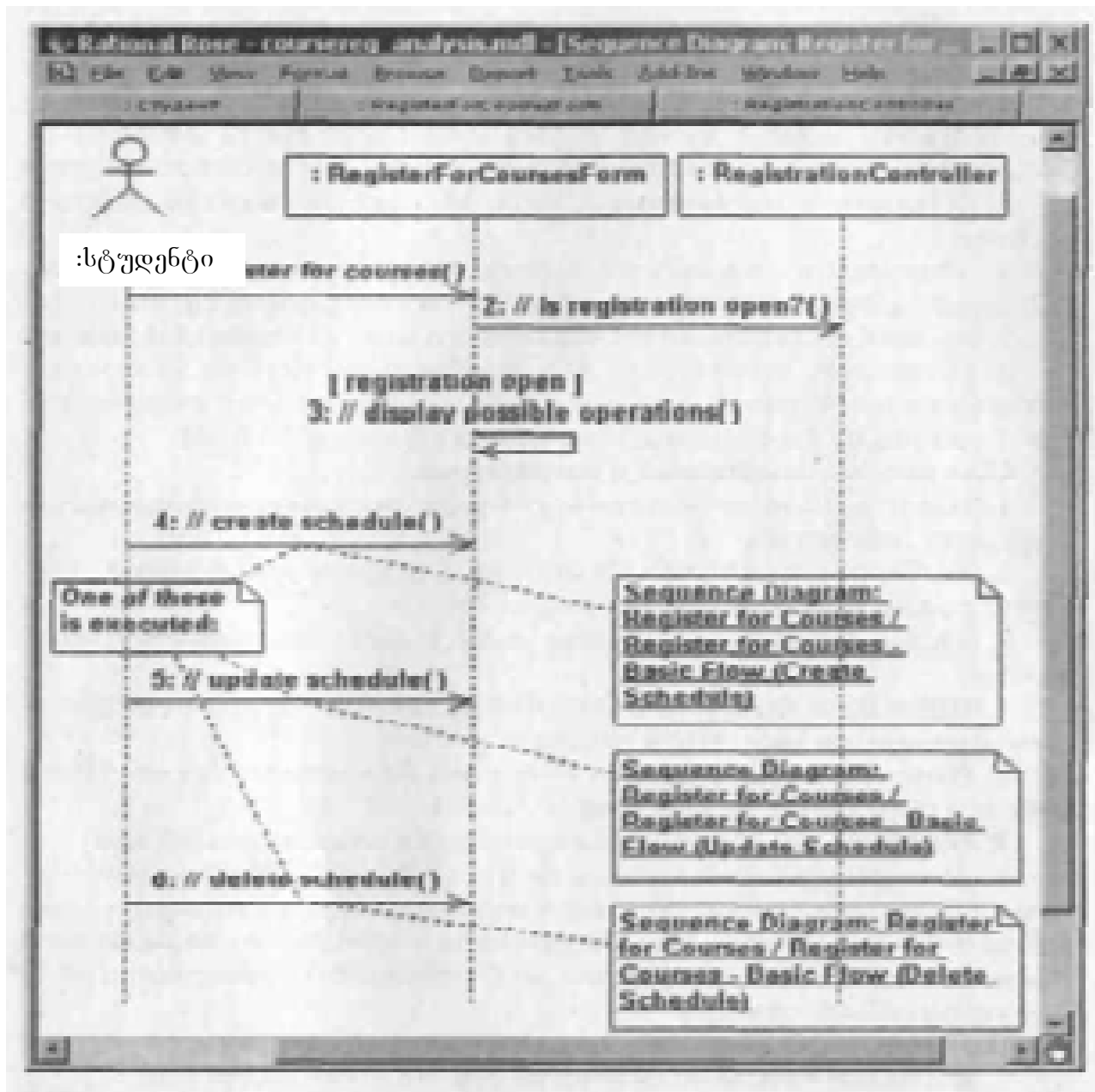
ნახ.4.4. მიმდევრობის დიაგრამა Register for Courses – Basic Flow.
