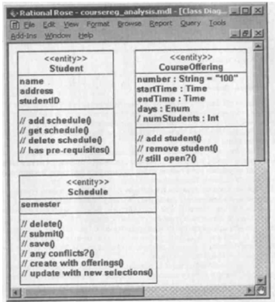
ნახ.4.10. “ანალიზის” კლასები ოპერაციებით და ატრიბუტებით
