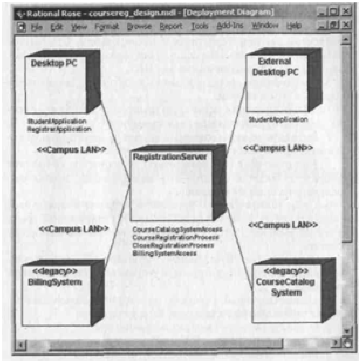
ნახ.5.10. რეგისტრაციის სისტემის ქსელური კონფიგურაცია პროცესების კვანძების მიხედვით განაწილებით
