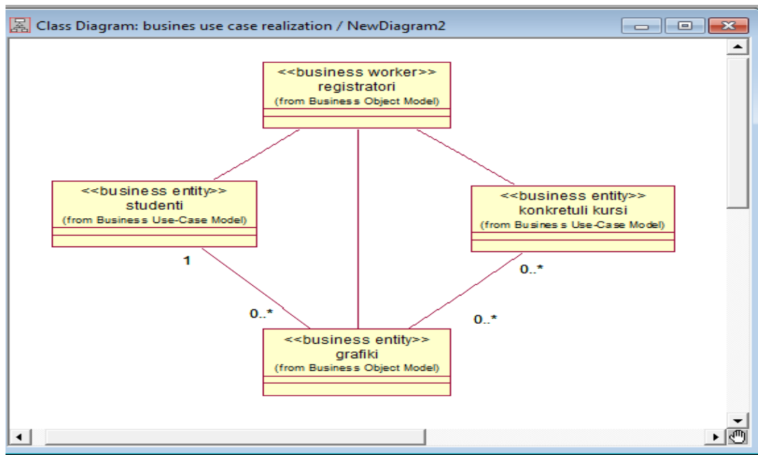
ნახ.2.2. ბიზნეს-ანალიზის მოდელის კლასების დიაგრამა
