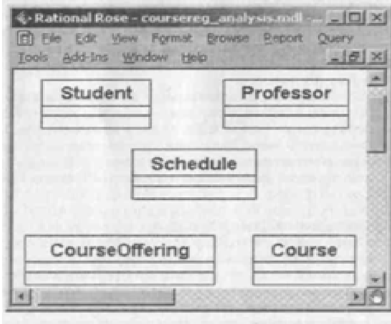
ნახ.4.2. რეგისტრაციის სიტემის ანალიზის კლასები
