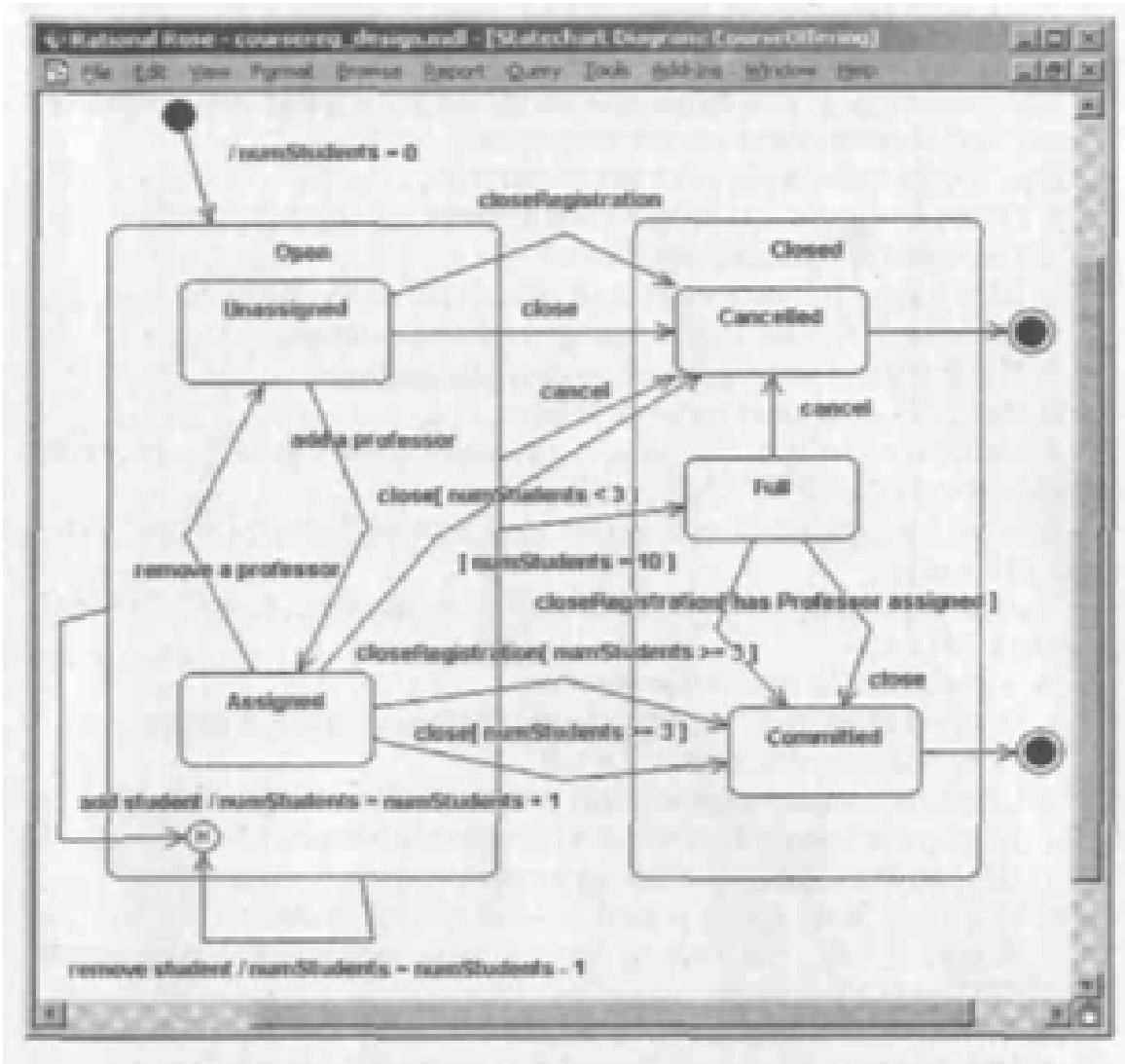
ნახ.5.13. მდგომარეობის დიაგრამა კომპოზიციური მდგომარეობებით
