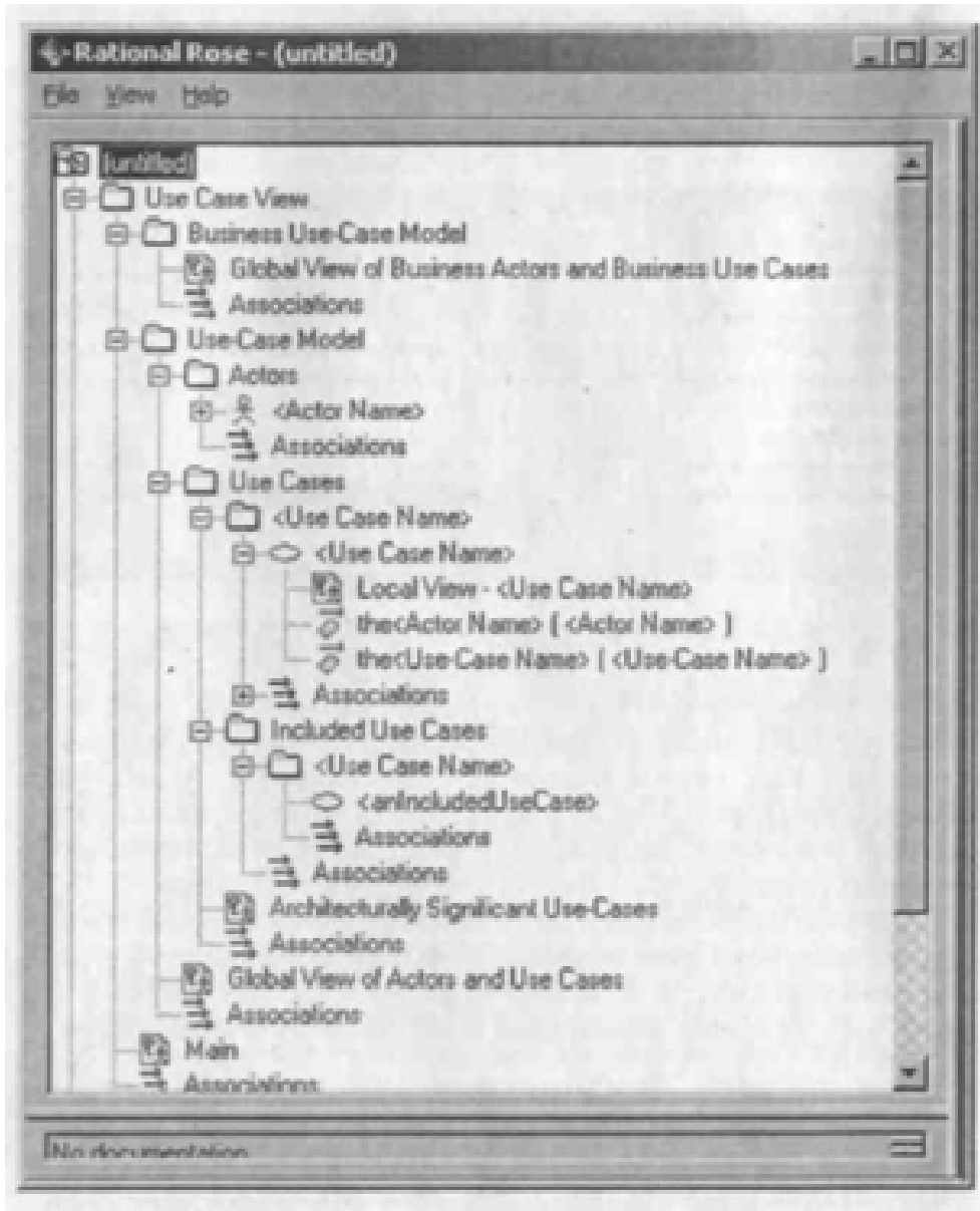
ნახ.1.2. გამოყენებით შემთხვევათა წარმოდგენა
