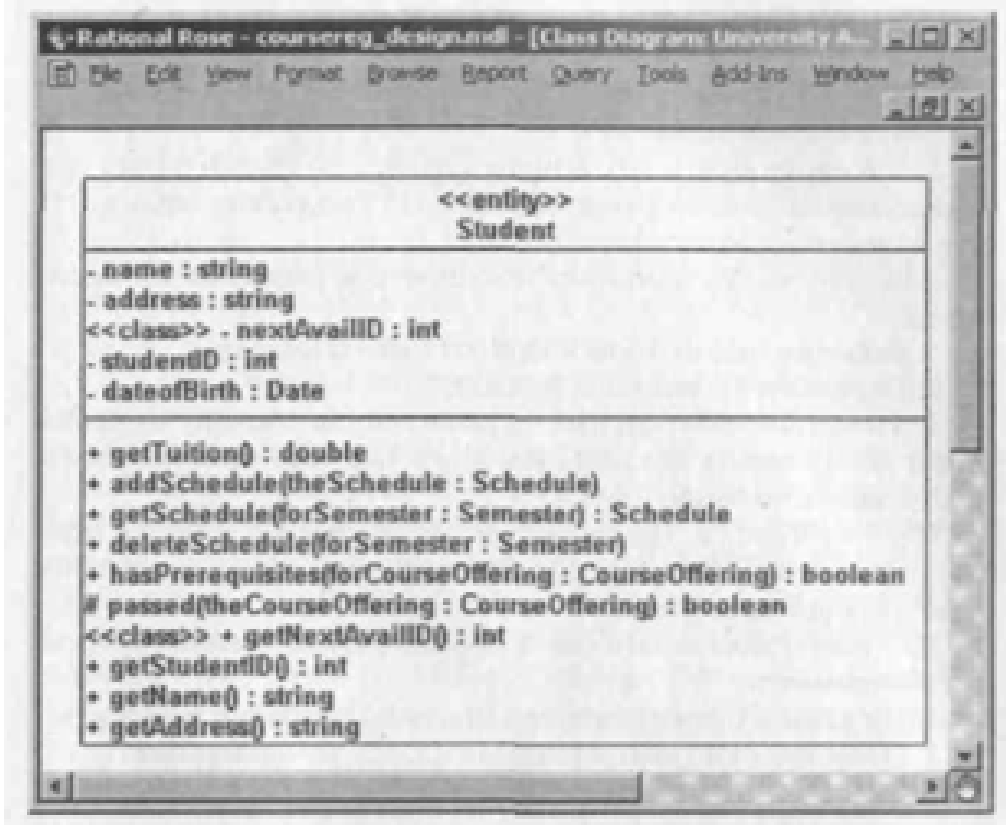
ნახ.5.11. კლასი Student ატრიბუტებითა და ოპერაციებით
