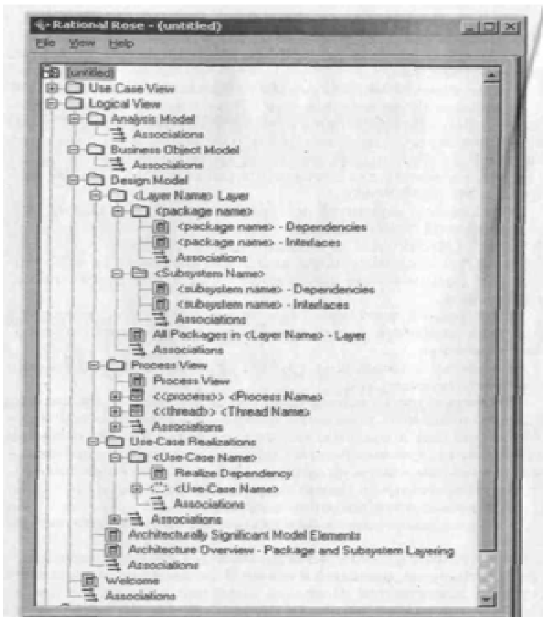
ნახ.1.3. ლოგიკური წარმოდგენა
