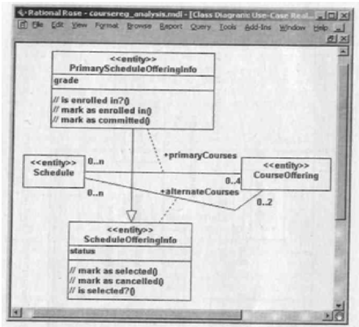
ნახ.4.12. დიაგრამა CourseOfferingInfo (ასოციაცია – კლასების მაგალითები)
