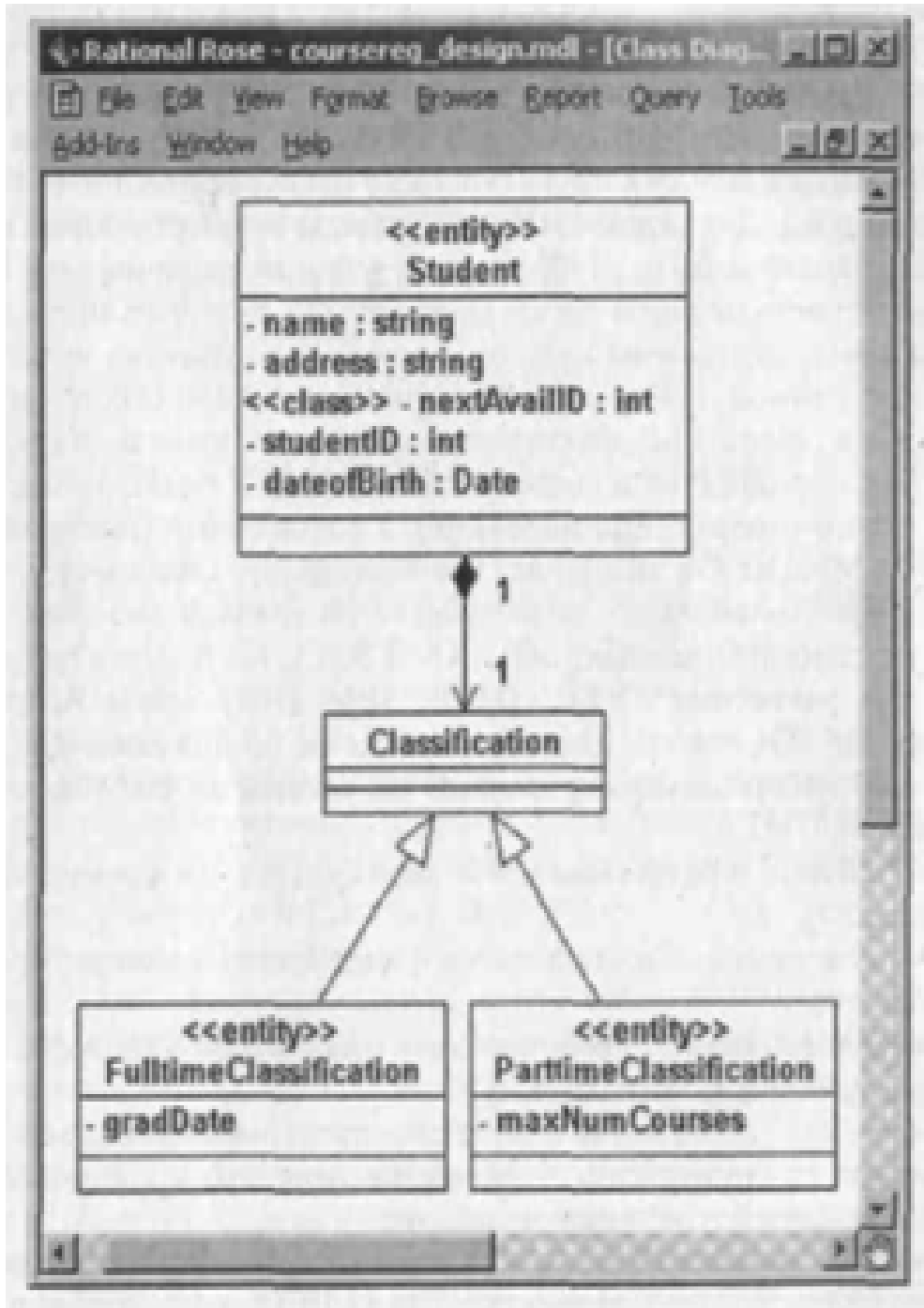
ნახ. 5.15. განზოგადების გარდაქმნა
