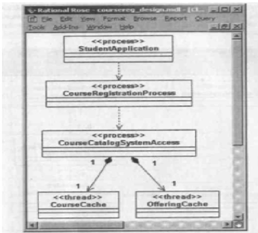
ნახ.5.6.პროცესები და ნაკადები
