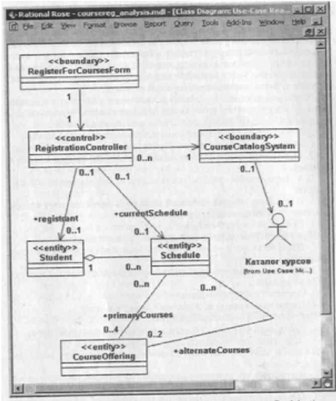
ნახ.4.13. კლასების მთლიანი დიაგრამა Register for Courses – Participating Classes (ატრიბუტების გარეშე)
