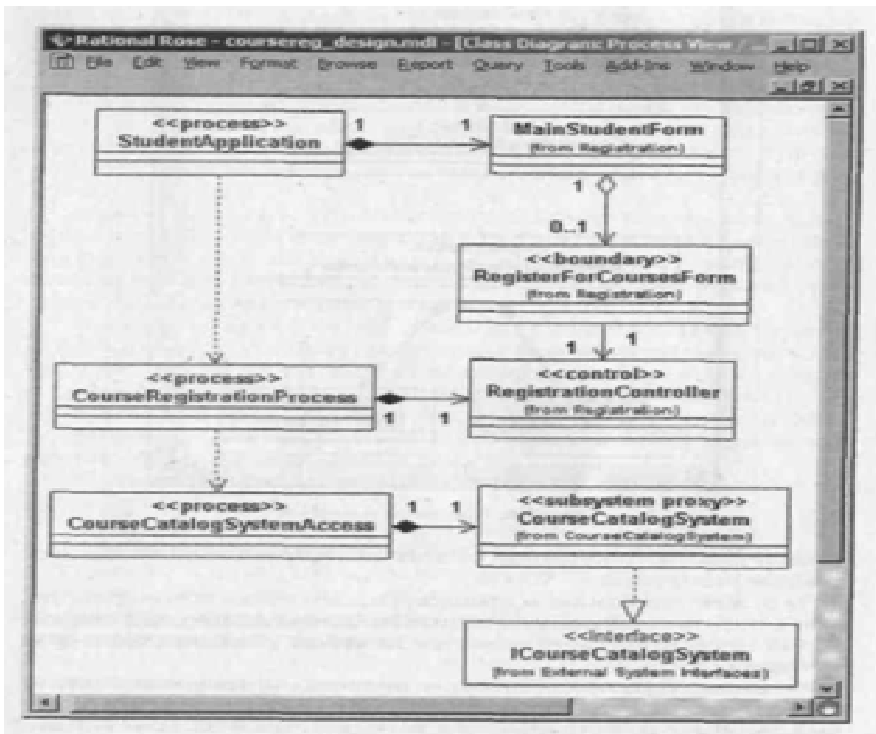
ნახ.5.7.კლასები, დაკავშირებულნი პროცესებთან
