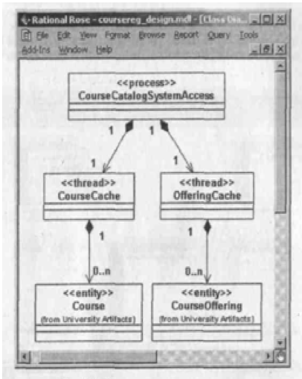
ნახ.5.8. კლასები, დაკავშირებულნი ნაკადებთან
