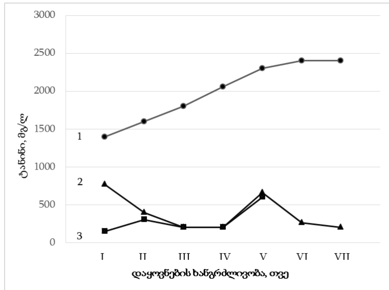
გრაფიკი 4. ყურძნის ტკბილის CO 2 -ის არეში(2) და CO 2 -ის წნევის ქვეშ(3), დურდოს CO 2 -ის არეში (1) დადულბულ და დავარგებულ ღვინომასალებში ტანინის შემცველობის დინამიკა დავარგების ხანგრძლივობისაგან დამოკიდებულებით
