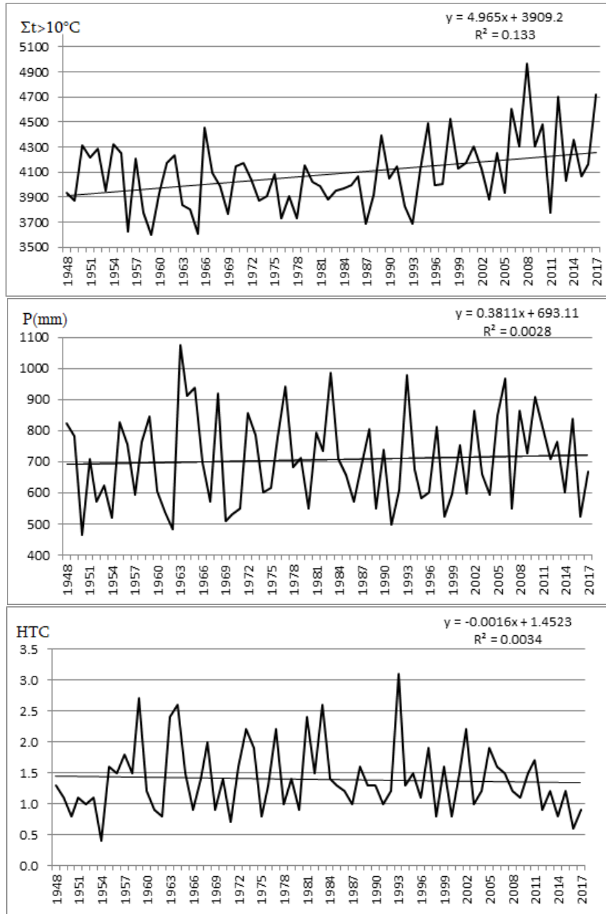
გრაფიკი 1. აქტიური ტემპერატურების ( >10^{\circ}\text{C} ), ატმოსფერული ნალექების (მმ) ჯამების და ჰოკ-ის მსვლელობის დინამიკა (ყვარელი)
