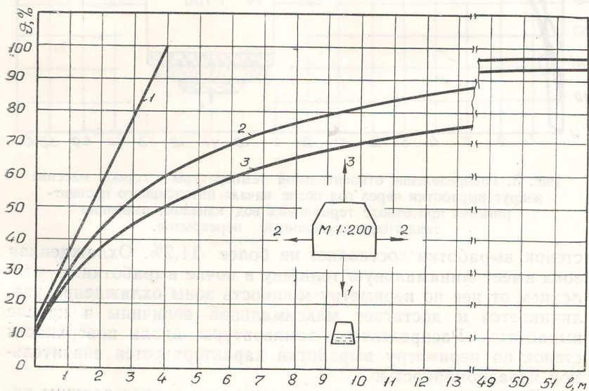
Рис. 2. Распределение относительной температуры в горном массиве вокруг выработки через 50 лет после начала интенсивного проветривания при отводе термальных вод специальной выработкой.
