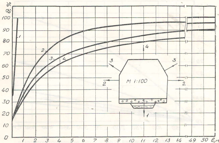
Рис. 6. Распределение относительной температуры в горном массиве вокруг выработки через 25 лет после вачала интенсивного проветривания при отводе термальных вод каналом с простым перекрытием.
