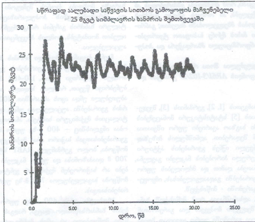
ნახ. 1. 25 მგვტ სიმძლავრის ხანძრის განვითარების დინამიკა
