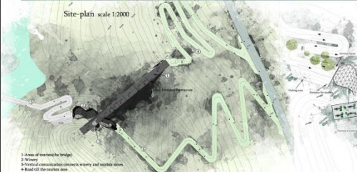
Site-plan scale 1:2000
