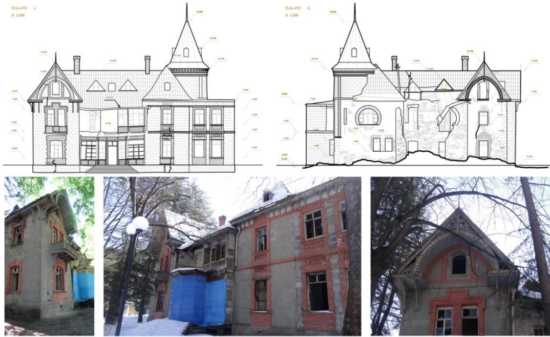
ნახ. 6. ძველი პოლიკლინიკის შენობის ფასადები, ნახაზები და ფოტოები, კოსტავას ბაღი, ბორჯომი
