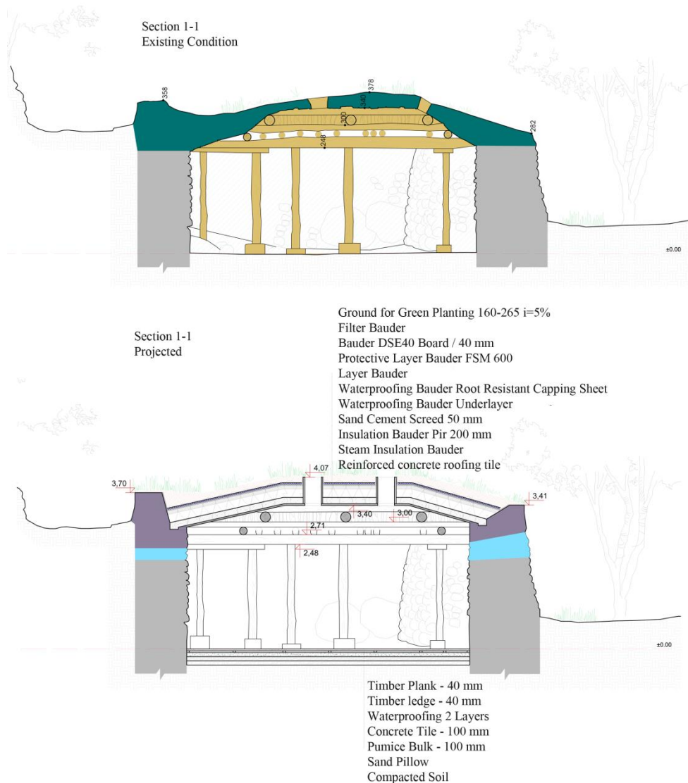
ნახ. 4: ჭაჭკარი. შენობის სექციები, არსებული და დაგეგმილი მდგომარეობა
